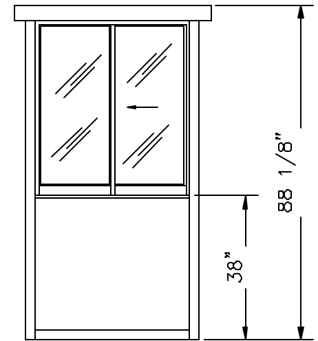
ELEVATION A
