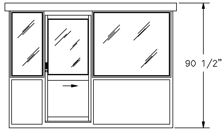
ELEVATION A
