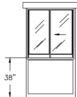
ELEVATION ②
