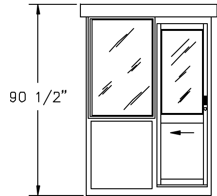
ELEVATION ①
