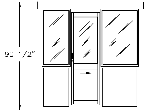
ELEVATION A
