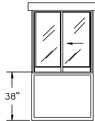
ELEVATION B
