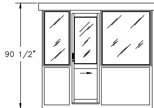
ELEVATION A
