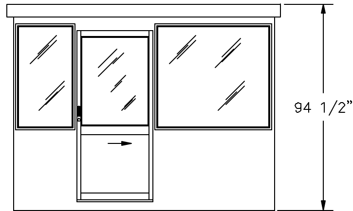
ELEVATION A
