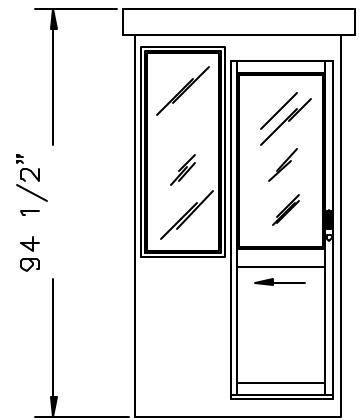
ELEVATION A
