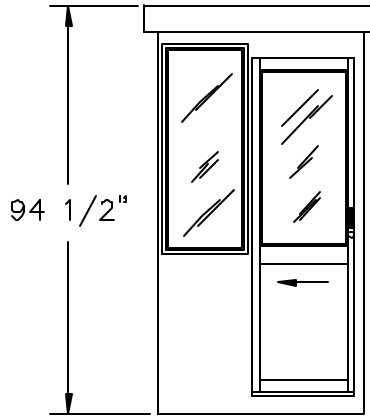
ELEVATION A
