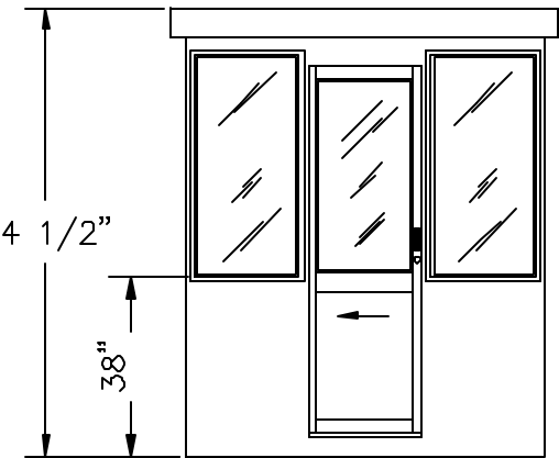
ELEVATION A
