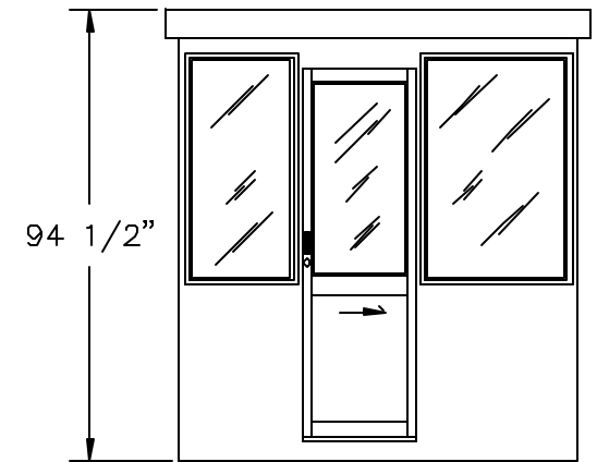
ELEVATION A
