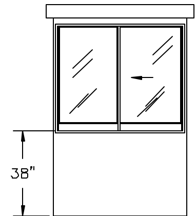
ELEVATION B
