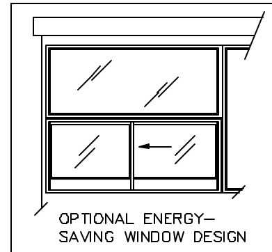
ELEVATION A
